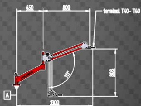
FIXATION AU BANC
